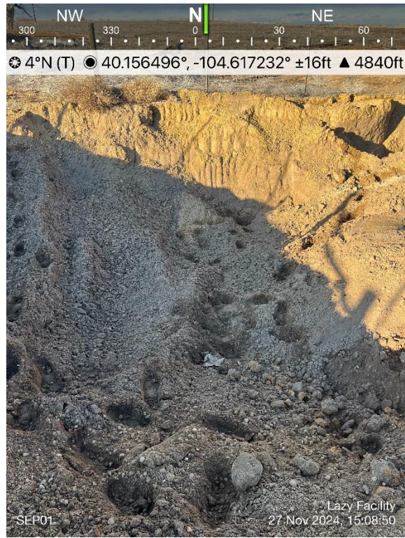
SEP01-RISER(2,4-12)@4'
