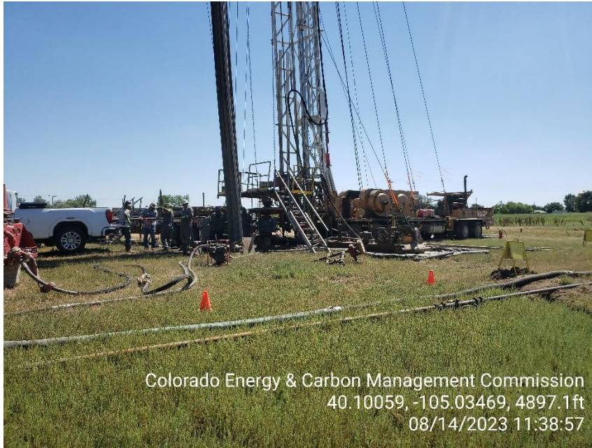
Photo 3 Rig.
