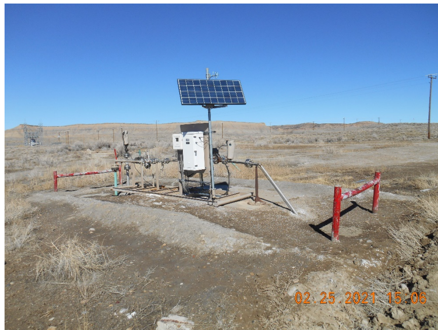
WAG skid
