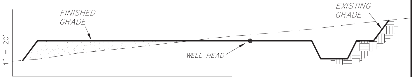
1" = 50' STA. 2+00
